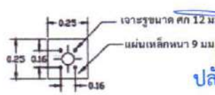
แบบขยายแผ่นเหล็กรับฐานราก มาตราส่วน 1:20
