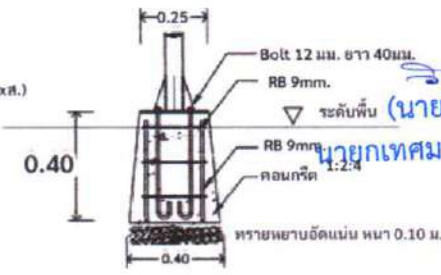
แบบขยายรูปตัดฐานราก มาตราส่วน 1:20
