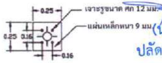
แบบขยายแผ่นเหล็กรับฐานราก มาตราส่วน 1:20
